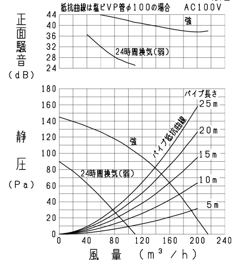
VD-15ZLPC 13 -IN/P-Q・騒音特性
