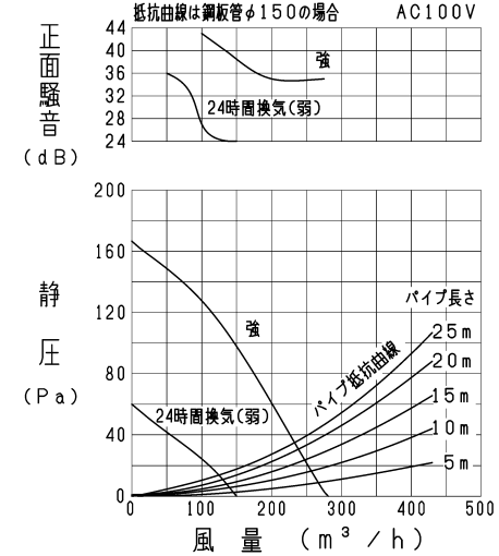
VD-18ZLX 13 -IN/P-Q・騒音特性
